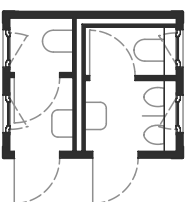
Damen-/Herren-WC Modell 1W315 2802x2438x2990
