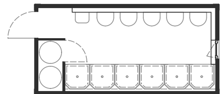
Duschen Modell 1Y622 2802x2990x6058
