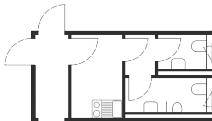
Küche-/WC-Kombination Modell 1K622 2802x2990x6058
