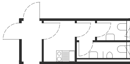
Küche-/WC-Kombination Modell 1K612 2802x2438x6058
