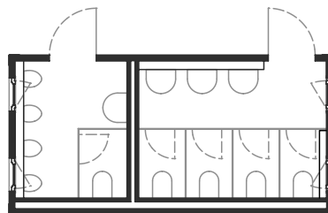
Damen-/Herren-WC Modell 1W6223 2802x2990x6058
