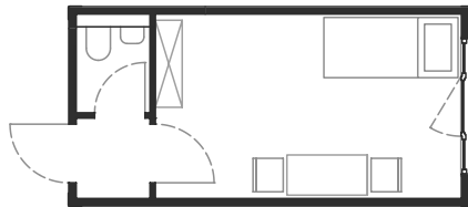
Modell 1L622 2802x2990x6058
