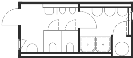
Dusch-/WC-Kombination Modell 1S622 2802x2990x6058
